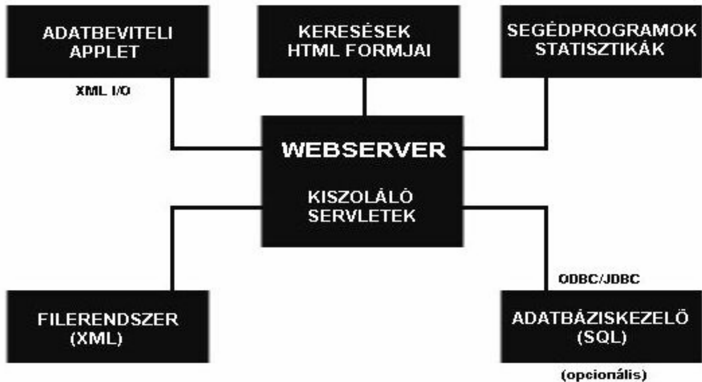
1. ábra Rendszerfelépítés
